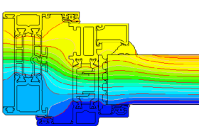
► 58BWST HI THERMAL PROFILE
