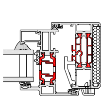
► 58BWST HI OPEN OUT CILL
