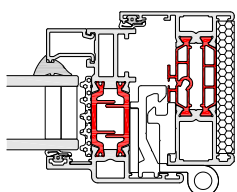
► 58BWST HI OPEN OUT HINGE JAMB
