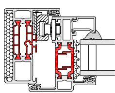
► 58BWST HI OPEN OUT LOCK JAMB
