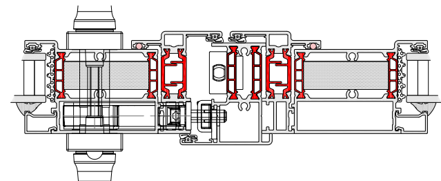
► 58BWST HI OPEN OUT LOCK JAMB
